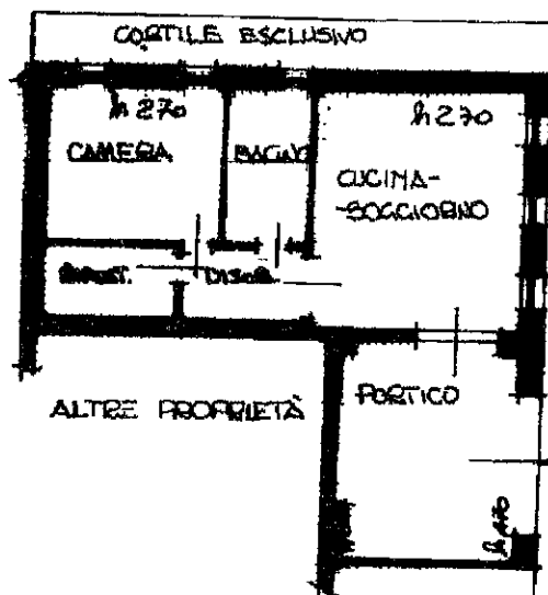
PIANTA PIANO TERRA (P.T.)
